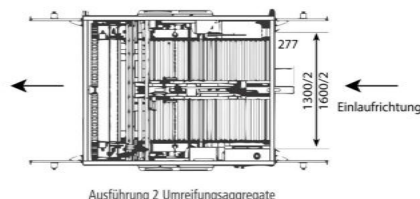
Ausführung 2 Umreifungsaggregat
