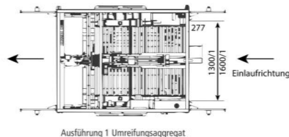
Ausführung 1 Umreifungsaggregat
